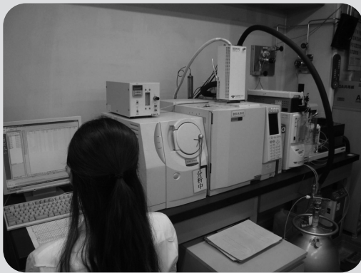
カビ臭物質の分析を行うバージ・トラップーガスクロマトグラフ質量分析計
